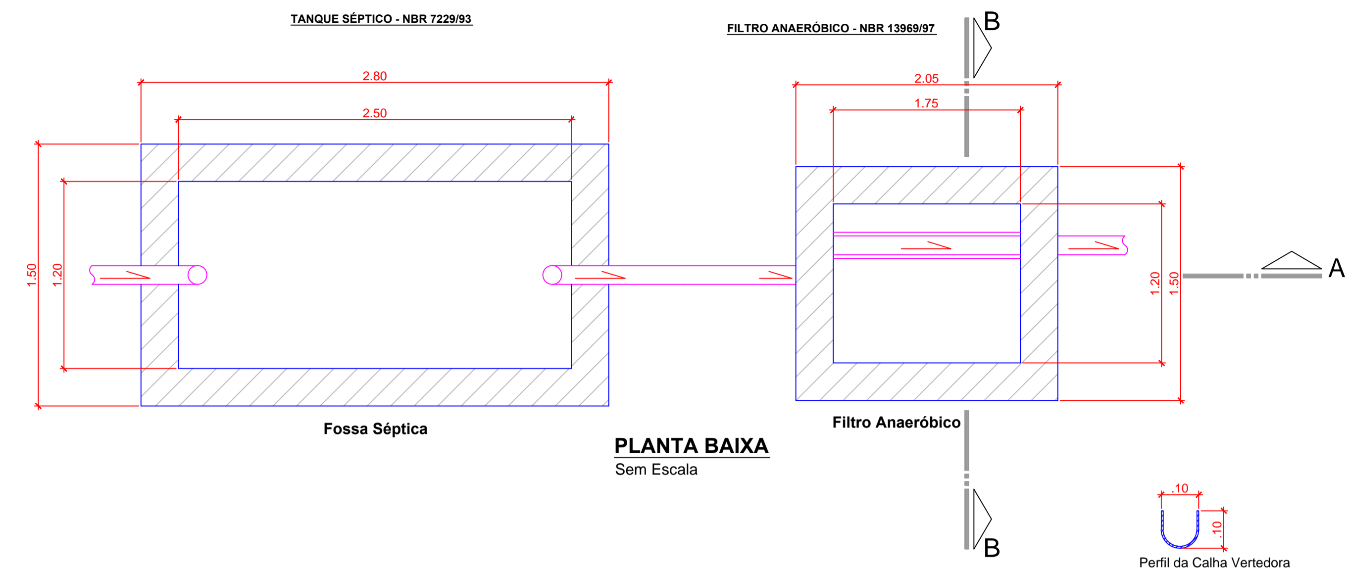
SISTEMA DE TRATAMENTO DE ESGOTO Sem Escala
